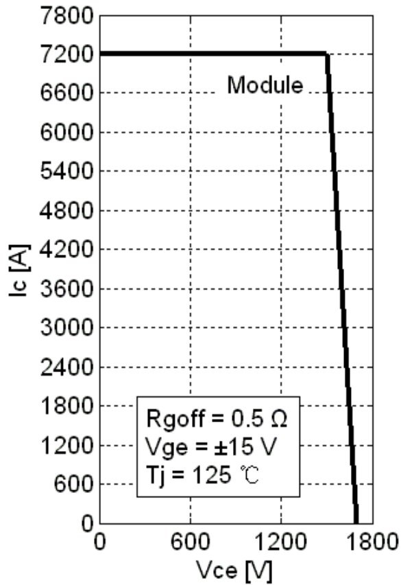
Fig 5. RBSOA
